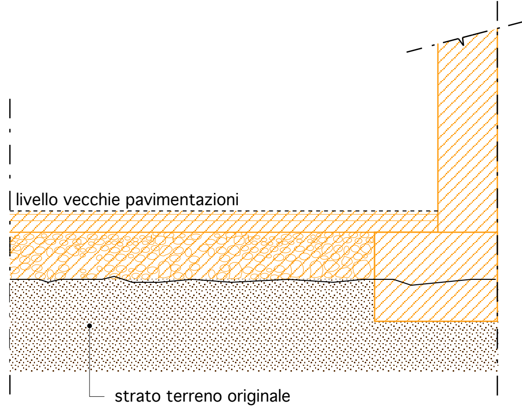
PARTICOLARE OPERE DI SISTEMAZIONE A TERRA SCALA 1/25
